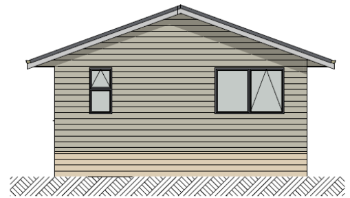
ELEVATION B
